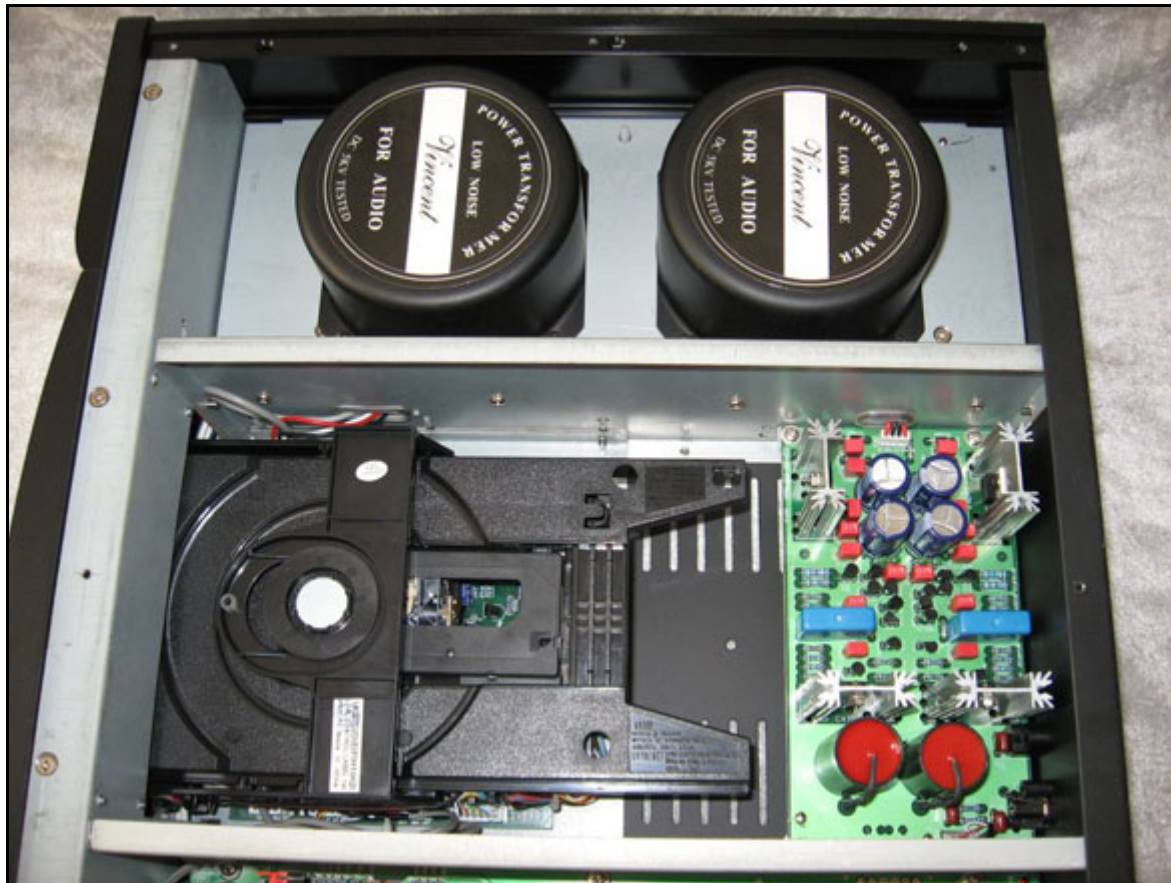
Strømforsyning og drev på Vincent CD-S5.
